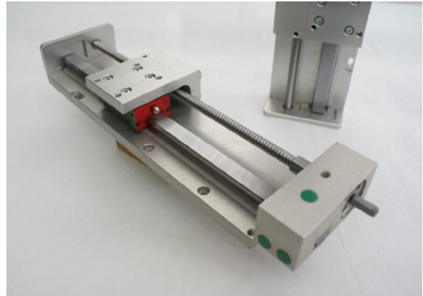
LINEARACHSE - mit Kugelgewinde antrieb
